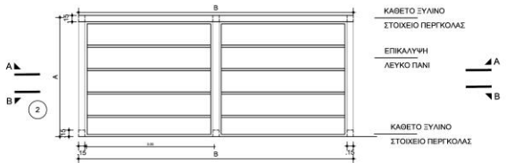
ΤΥΠΟΣ Α - ΕΛΕΥΘΕΡΗ ΤΟΠΟΘΕΤΗΣΗ
